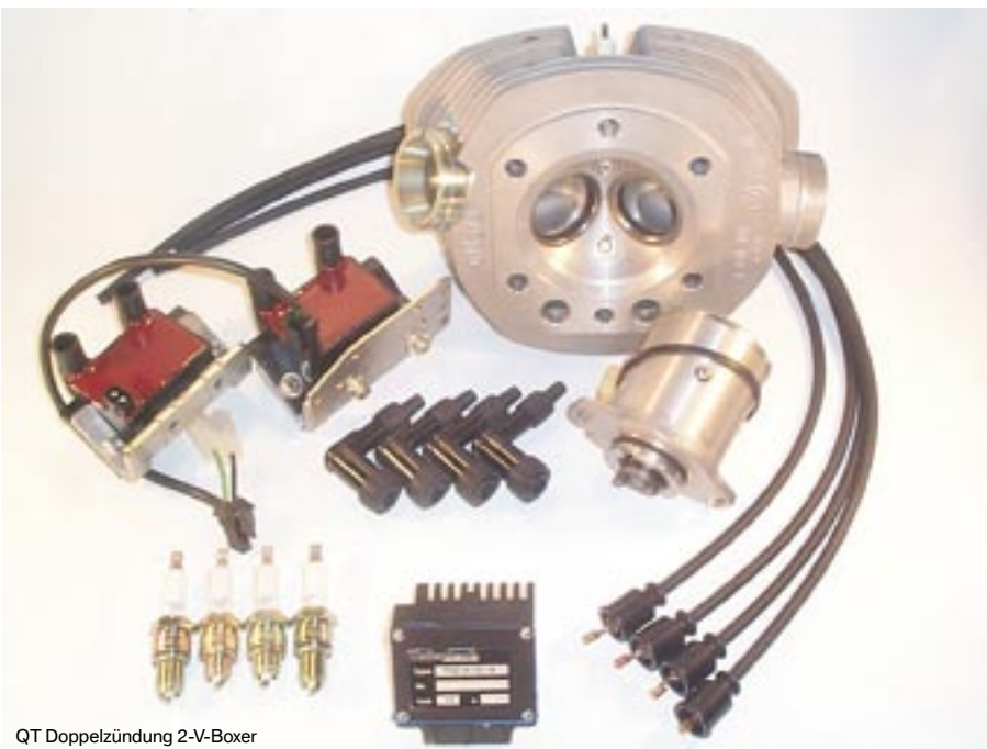
QT Doppelzündung 2-V-Boxer
